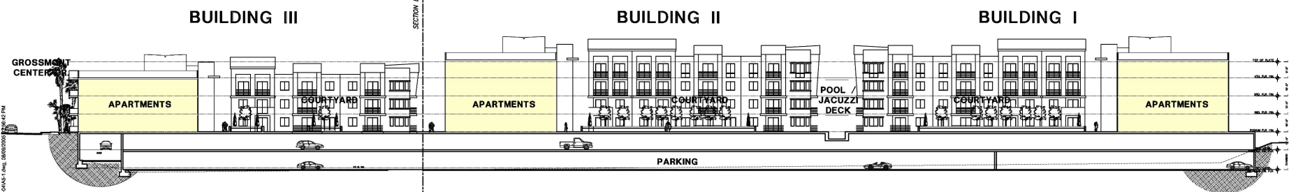
EAST PARCEL LONGITUDINAL SECTION "A-A"
